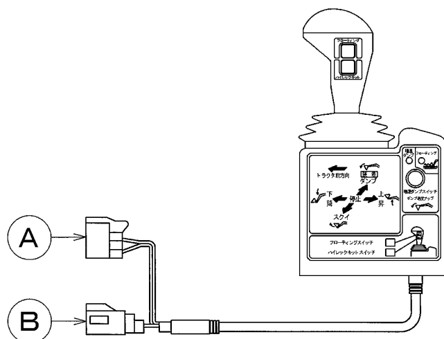
8 極コネクタ ( から見た図 )
